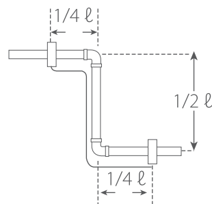
Pieza en forma de S
