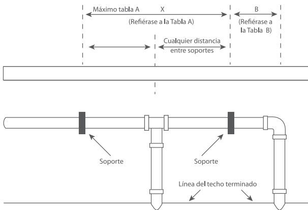
Separación entre soportes para codos y tubos en T
