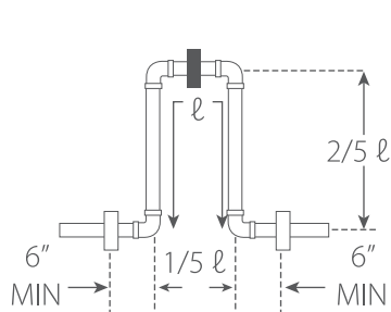
Tubería en curva cerrada
